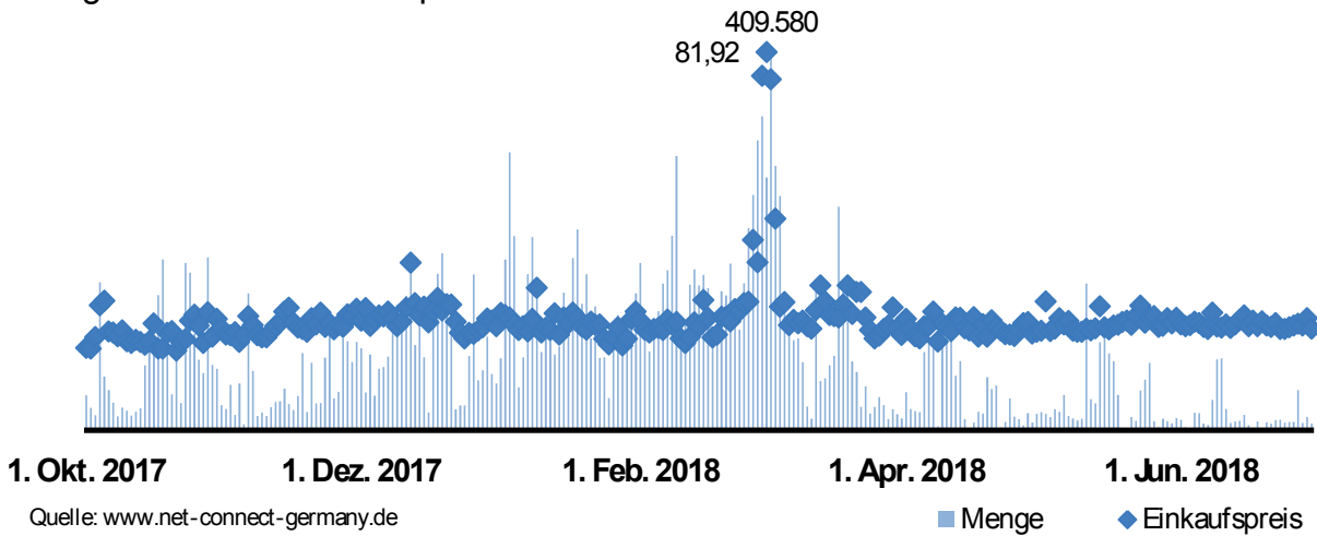
Abbildung 4: Externe Regelenergiekaufpreise und -mengen ab 1. Oktober 2017 für MOL 2 im Marktgebiet NetConnect Germany, Stand Juli 2018
