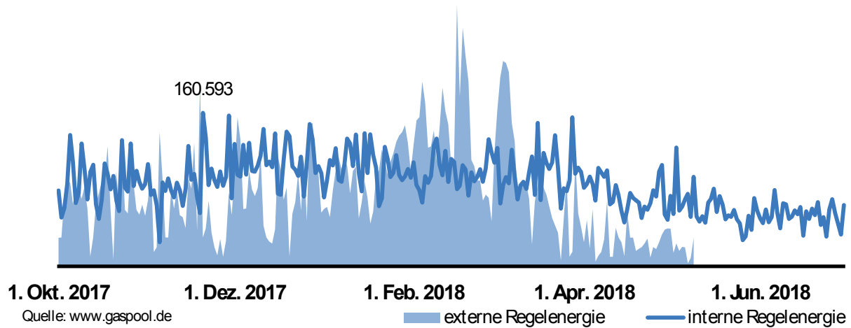
Abbildung 2: Regelenergieeinsatz ab 1. Oktober 2017 bei Gaspool, Stand Juli 2018
