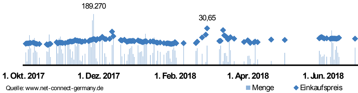
Abbildung 3: Externe Regelenergiekaufpreise und -mengen ab 1. Oktober 2017 für MOL 1 im Marktgebiet NetConnect Germany, Stand Juli 2018
