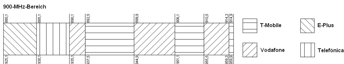
Abbildung 1: Lage der Frequenzzuteilungen im 900-MHz-Band
